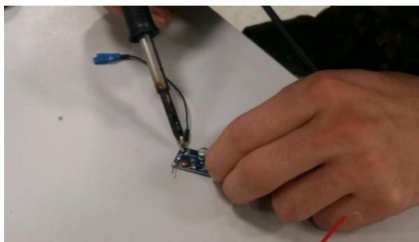
Рис. 9. Пайка проводов к входам и выходам DC-DC повышающих преобразователей
