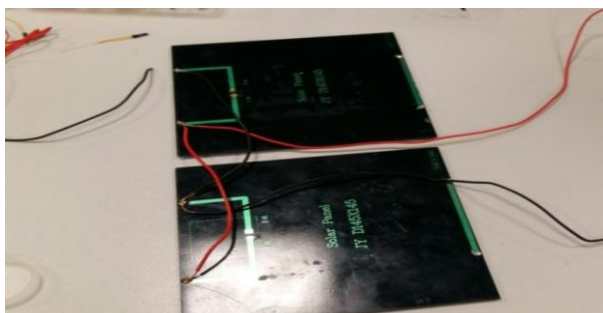
Рис. 8. Пайка проводов к полюсам солнечных панелей
