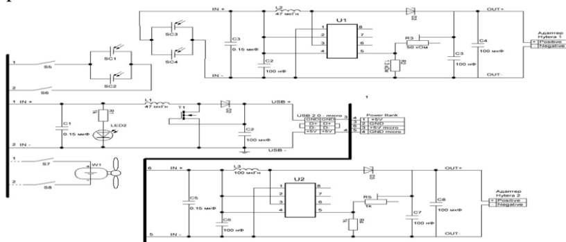
Рис. 2. Электрическая принципиальная схема зарядного устройства на альтернативных источниках энергии (ветрогенератор и солнечные панели)
