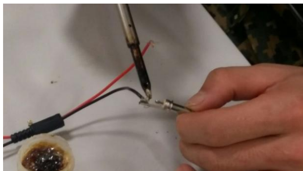
Рис. 7. Пайка провода к штекеру
